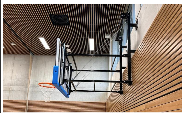
Basketballwandanlage elektrisch hochklappbar und höhenverstellbar (Art.-Nr. 36017+36018)
