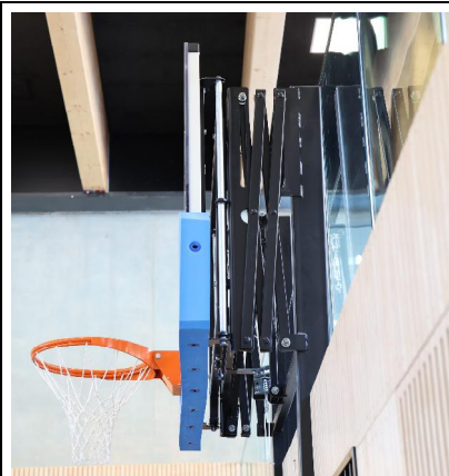
Wandgerüst mit Scherenmechanismus (Art.-Nr. 36080+36081+36082+36083)
