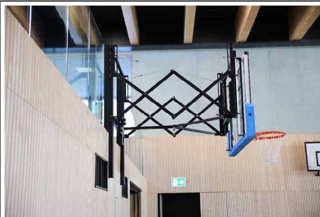
Wandgerüst mit Scherenmechanismus (Art.-Nr. 36080+36081+36082+36083)
