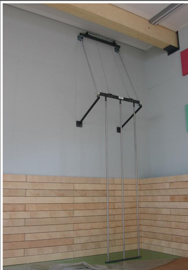
Kletterstangen elektrisch hochziehbar (Beispiel 3fach) - Nutzungsstellung
