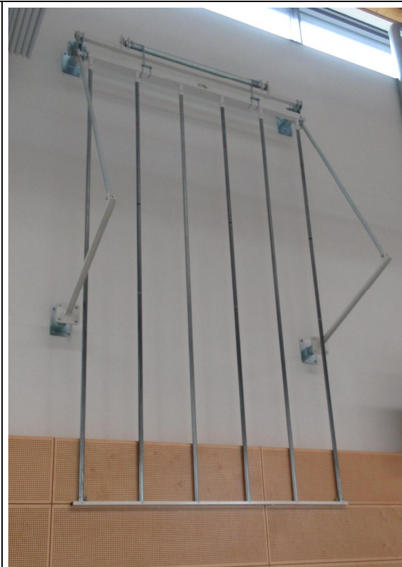
Kletterstangen elektrisch hochziehbar (Beispiel 6fach) - Parkstellung
