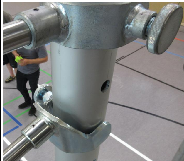
Recksäule Artikel-Nr. 80060 mit beispielhaft Reckstange Artikel-Nr. 80030
