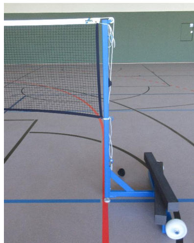
37200 Badminton-Anlage freistehend, fahrbar, mit 2 x 37201 Zusatzgewichte(zur Wettkampfnutzung)
